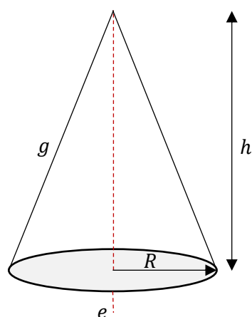
CONE RETO
