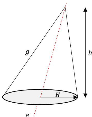
CONE OBLÍQUO
