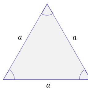
EQUILÁTERO
